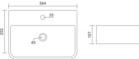
GEM L 252 W 364 H 107mm L 10" W 15" H 4"
