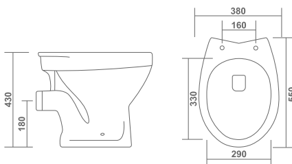
EWC - P L 550 W 380 H 430mm
