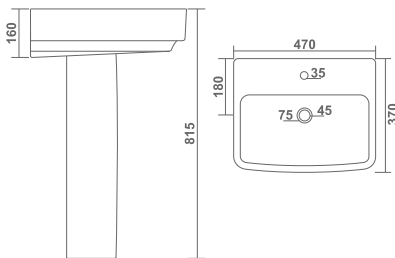
MINI VOLVO SET L 370 W 470 H 815mm L 15" W 19" H 33"
