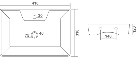
PLAZMA L 310 W 410 H 120mm L 12" W 16" H 5"
