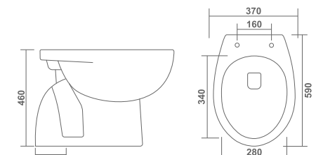
OZONE L 590 W 370 H 460mm
