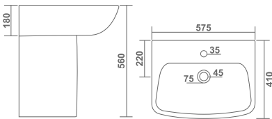
L 410 W 575 H 560mm L 16" W 23" H 22"
